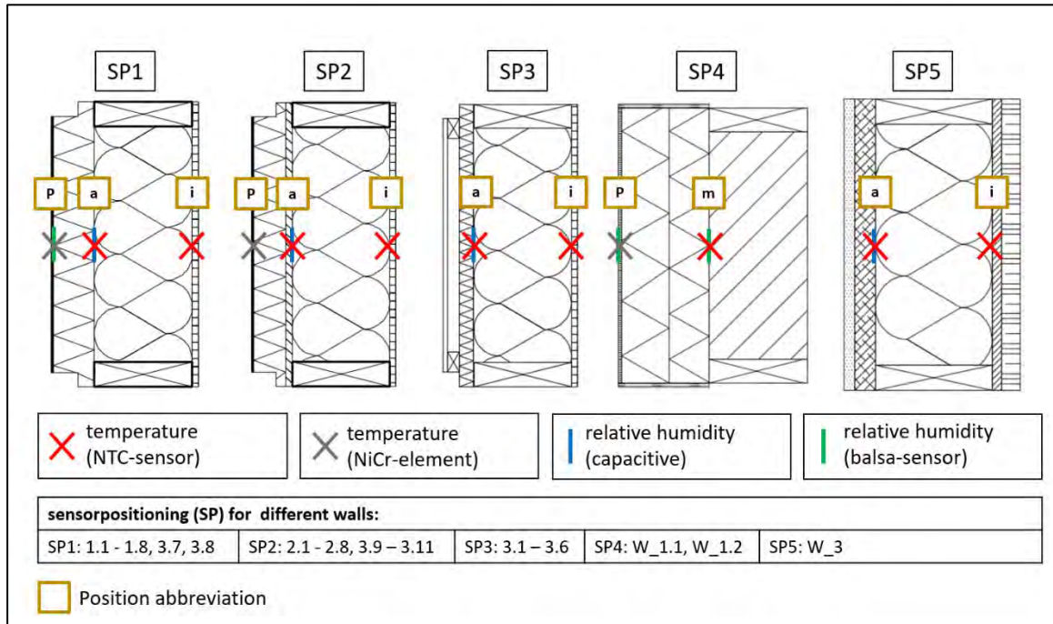
Abbildung 15: Übersicht zu den Sensorpositionen und -arten im Bauteilquerschnitt. Angaben zu entsprechenden Wandelementnummern und Positions Kürzeln.
