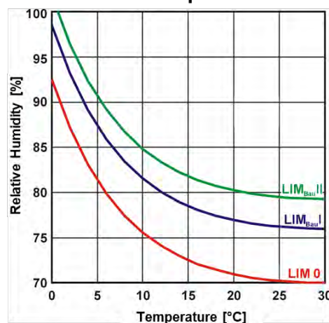
Abbildung 33: Sorptionsisotherme (oben links) und Diffusionswiderstand der Sporenwand (oben rechts) der Modell-Pilzspore des Schimmelpilz-Prognosemodells WUFI® Bio. Die Grenzkurven „Lowest Isopleth for Mould“ für je nach Nährstoffangebot unterschiedlich anfällige Materialien (Klasse 0 für optimalen Nährboden und die Klassen Bau I und Bau II für biologisch verwertbare bzw. nicht verwertbare Baustoffe).
