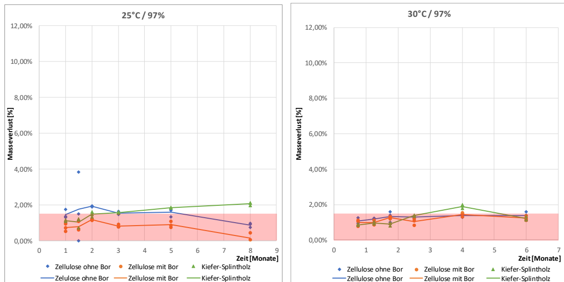
Abbildung 1: Masseverluste der Probekörper; Inkubation bei 25 °C und 30 °C sowie 97 % r.F. (transparent rot markiert = Bereich der Messungenauigkeit von 1,5 M.-%)
