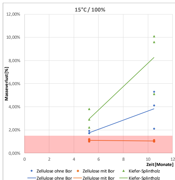
Abbildung 2: Masseverluste der Probekörper; Inkubation bei 15 °C und 100 % r.F. (transparent rot markiert = Bereich der Messungenauigkeit von 1,5 M.-%)
