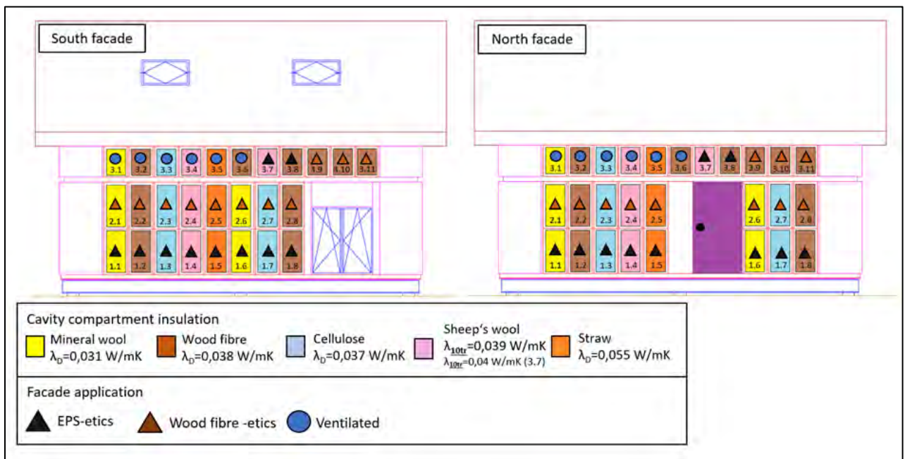
Abbildung 4: Fassadenansichten Süd- und Nord mit Elementnummern sowie Gefachdämmungs- und Fassadenausführungen.
