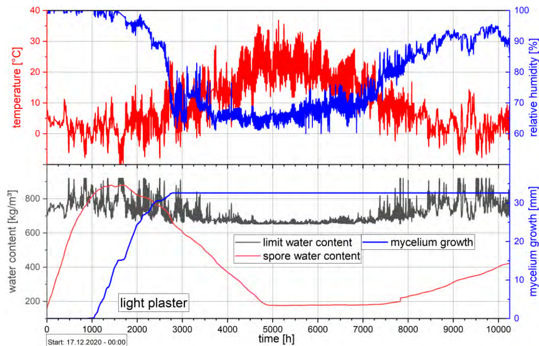
Abbildung 40: Temperatur und relative Luftfeuchte am hydrophobierten Holzfaser-WDVS (Messwerte) aus dem Trocken verfahren (Dichte lt. Datenblatt: 140 kg/m³) unterhalb des hellen Putzes über den gesamten Messzeitraum (oben). Parallel dazu: Aus Temperatur abgeleiteter Grenzwassergehalt (Isoplethenmodell: ThermNat II), Entwicklung des instationär hergeleiteten Sporenwassergehalts und resultierendes Sporenwachstum (unten).
