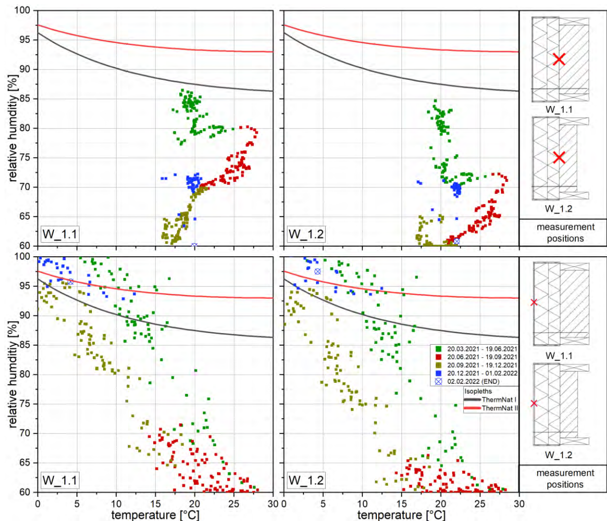
Abbildung 51: Temperatur-/Luftfeuchtekombinationen (24h-Mittel der Messwerte) am WDVS aus hydrophobierter Holzfaser aus dem Trockenverfahren (Dichte lt. Datenblatt: 110 kg/m 3 ) unterhalb der Putzschicht (Messposition P – unten) sowie im Bauteilinneren (Messposition m – oben) für die Varianten auf 25 cm (links) und 15 cm (rechts) starken Kalksandsteinmauerwerk auf der Westfassade.
