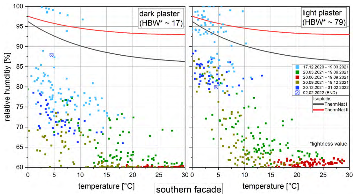
Abbildung 46: Temperatur-/Luftfeuchtekombinationen (24h-Mittel der Messwerte) am WDVS aus hydrophobierter Holzfaser aus dem Trockenverfahren (Dichte lt. Datenblatt: 140 kg/m 3 ) unterhalb der Putzschicht (Messposition P) für die Varianten mit dunkler (links) und heller (rechts) Putzfarbe auf der Nordfassade. Dargestellt sind die Messwerte der Variante S 2.6 (links) und die arithmetischen Mittelwerte über die Varianten S 2.1 bis N 2.5 (rechts)
