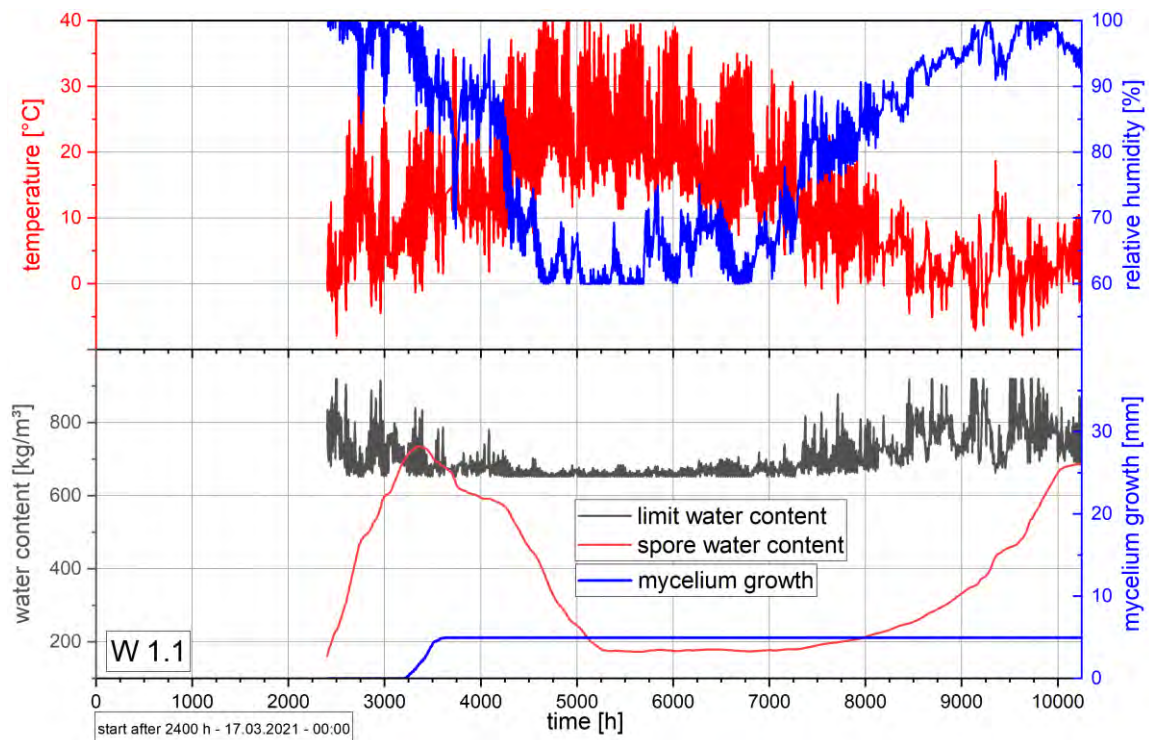
Abbildung 52: Temperatur und relative Luftfeuchte am WDVS aus hydrophobierter Holzfaser aus dem Trockenverfahren (Dichte lt. Datenblatt: 110 \text{ kg/m}^3 ) unterhalb der Putzschicht (Messposition P) für die Variante auf 25 cm starken Kalksandsteinmauerwerk auf der Westfassade (oben). Parallel dazu: Aus Temperatur abgeleiteter Grenzwassergehalt (Isoplethenmodell: ThermNat II), Entwicklung des instationär hergeleiteten Sporenwassergehalts und resultierendes Sporenwachstum (unten).
