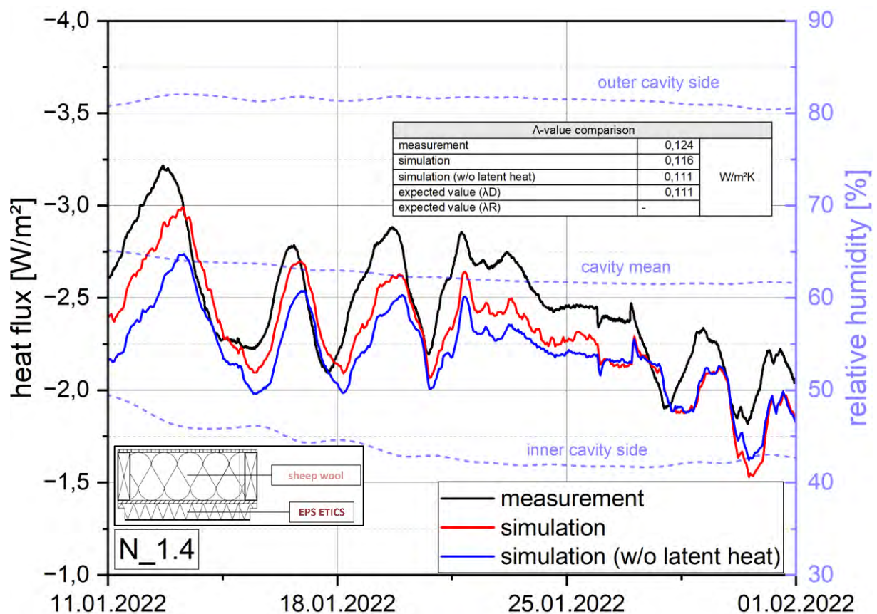
Abbildung 62: Abgleich zwischen den gemessenen und simulierten Wärmeströmen (24h Mittelwert, gleitend) des Aufbaus mit Schafwoll- und EPS WDV (N 1.4), sowie das Luftfeuchteniveau an verschiedenen Stellen im Gefach. Tabellarische Auflistung der durchschnittlichen dynamischen Wärmedurchlasskoeffizienten ( \Lambda_{\text{dyn}} ) im Mess- bzw. Simulationszeitraum sowie deren für den betrachteten Zeitraum berechneten Erwartungswert auf Basis der Herstellerangaben zum Nennwert ( \Lambda_D ) der Dämmstoffe.
