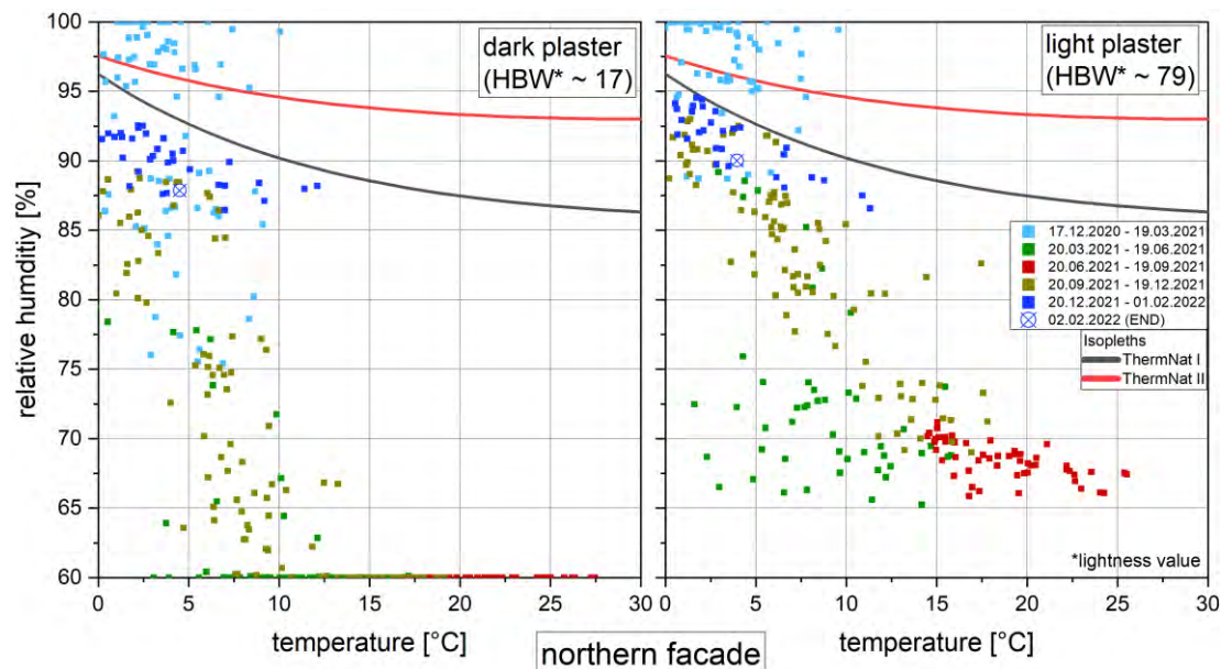
Abbildung 39: Temperatur-/Luftfeuchtekombinationen (24h-Mittel der Messwerte) am hydrophobierten Holzfaser-WDVS aus dem Trockenverfahren (Dichte lt. Datenblatt: 140 kg/m 3 ) unterhalb der Putzschicht (Messposition „P“) für die Varianten mit dunkler (links) und heller (rechts) Putzfarbe auf der Nordfassade. Dargestellt sind die arithmetischen Mittelwerte der Messungen über die Varianten N 2.6 und N 2.7 (links) und die Varianten N 2.1 bis N 2.5 (rechts).
