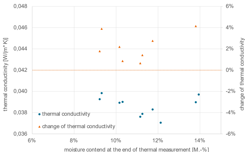
Abbildung 75: Gemessene und auf 10 °C umgerechnete feuchte Wärmeleitfähigkeit (blaue Punkte) für die einzelnen Schichten bezogen auf den Feuchtegehalt. Änderung der Wärmeleitfähigkeit (orangene Dreiecke) bezogen auf die vorher bestimmte trockene Wärmeleitfähigkeit.
