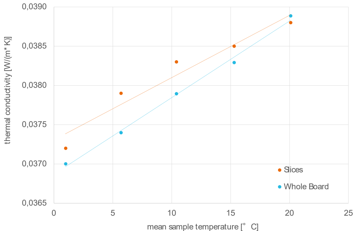
Abbildung 70: Gemessene Temperaturabhängigkeit der Wärmeleitfähigkeit der getrockneten Proben als einzelne Messpunkte und lineare Regressionsgeraden für die komplette und die geschichtete Platte jeweils mit Angabe der mathematischen Gleichung.
