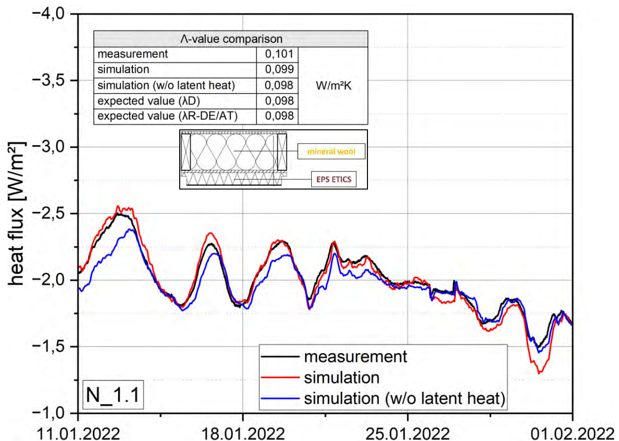
Abbildung 56: Abgleich zwischen den gemessenen und simulierten Wärmeströmen (24h Mittelwert, gleitend) des Aufbaus mit Mineralwollgefachdämmung und EPS WDV (N 1.1). Tabellarische Auflistung der durchschnittlichen dynamischen Wärmedurchlasskoeffizienten ( \lambda_{dyn} ) im Mess- bzw. Simulationszeitraum sowie deren für den betrachteten Zeitraum berechneten Erwartungswert auf Basis der Herstellerangaben zu Nenn- ( \lambda_D ) und Bemessungswerten ( \lambda_r ) der Dämmstoffe.
